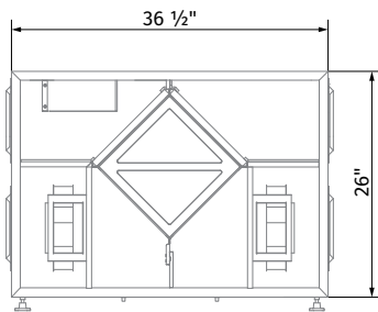
BLAULITE ERV 5 / ERV 8 / ERV 13 / ERV 17 / ERV 25
